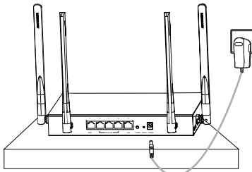
图5-2 电源连接示意图
